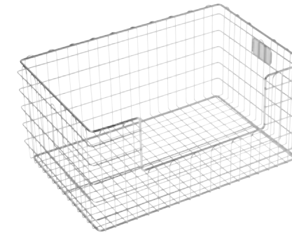
Grand panier 60 x 30 x 30 cm Réf : 805040
